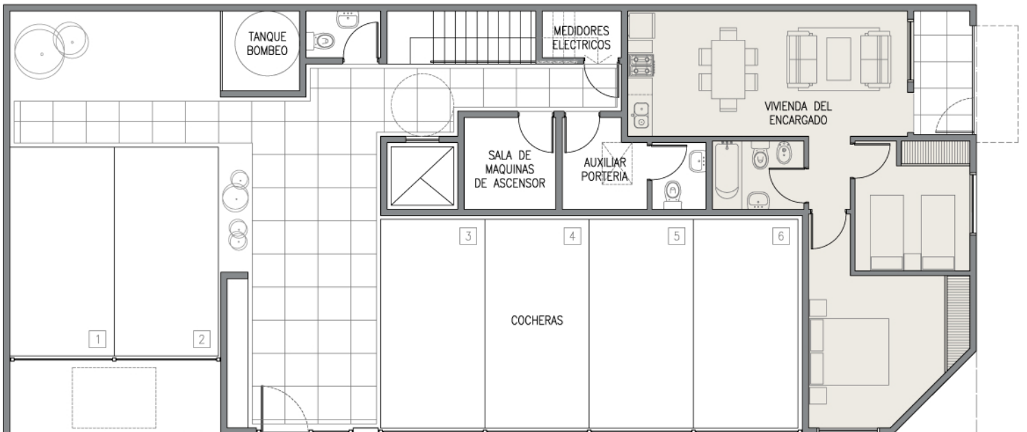
PLANTA BAJA
