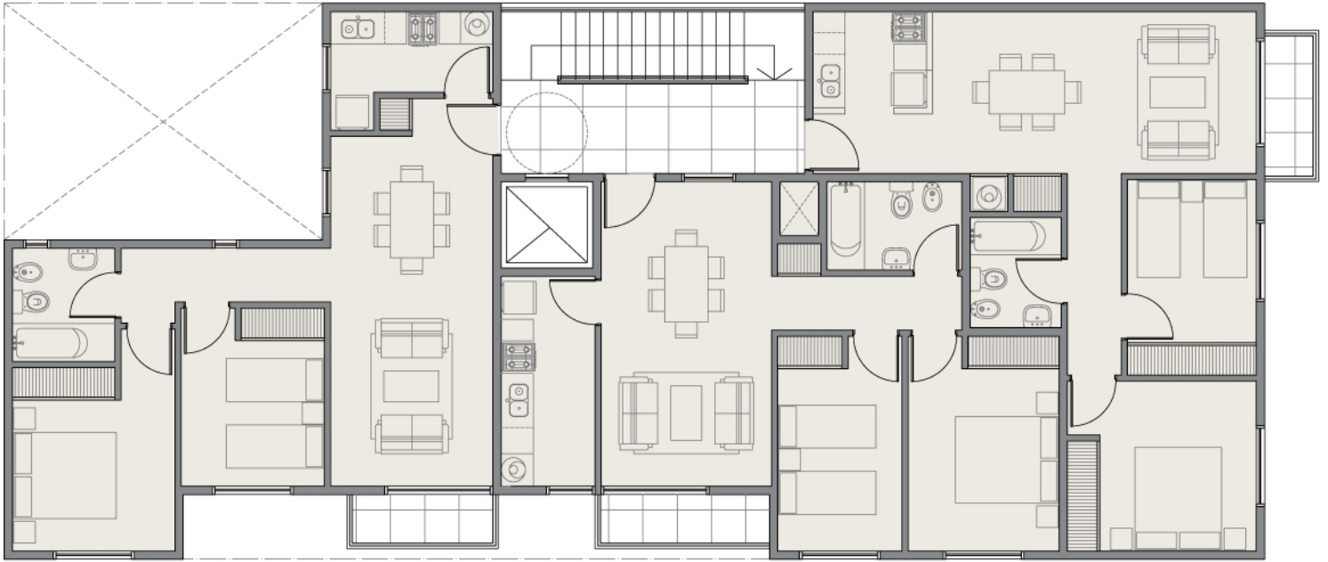
PLANTA 1° A 4° PISO
